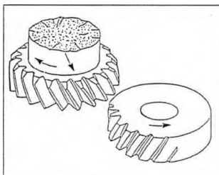
Bild iv.2.1 wälzstoßen einer Schrägverzahnung vom Schrägungswinkel der Verzahnung,
